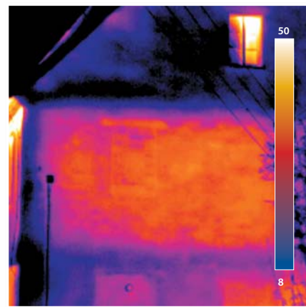
Дефект изоляции
