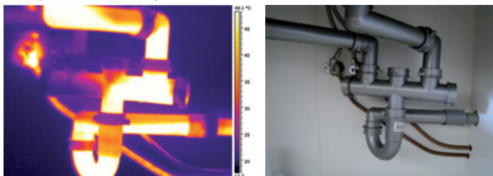
Тепловидение помогает находить неполадки в трубах.
