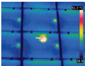
Эта горячая точка в солнечном фотоэлементе говорит о его повреждении.
