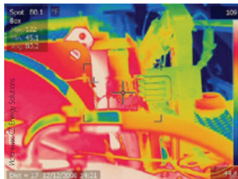
Исследование трансмиссии ветровой турбины с использованием термических изображений. Проверка проводилась на высоте около 50 метров.
