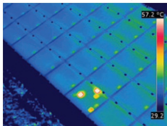
На этом термическом изображении виден так называемый лоскутный рисунок, который говорит о наличии в панели дефектного шунтирующего диода.
