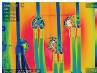
Тепловизионные камеры также можно использовать для полной проверки системы, частью которой являются ветровые турбины. Один из этих трехфазных разъемов (крайний правый) значительно теплее остальных. Этот дефект был локализован и исправлен до того, как возникла неисправность.
