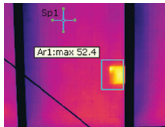
На этом термическом изображении показан горячий участок, возникший вследствие разрушения фотоэлемента в стандартном модуле на 60 элементов.
