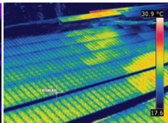
На этом термическом изображении видны обширные участки с повышенной температурой. Без дополнительной информации сложно сказать, являются ли они тепловыми аномалиями либо вызваны тенью или отражением.
