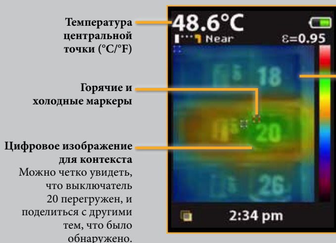
Накладываемая ИК тепловая карта
